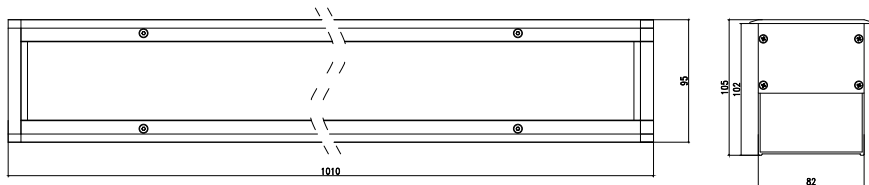
开孔尺寸: L1005*W85*H105mm ±1mm
